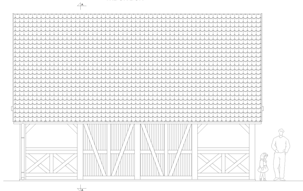
WIDOK BOK
