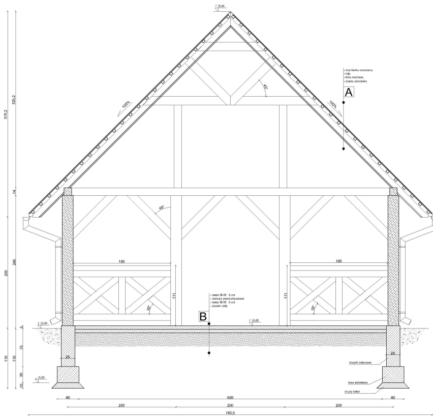
PRZEKRÓJ A-A
