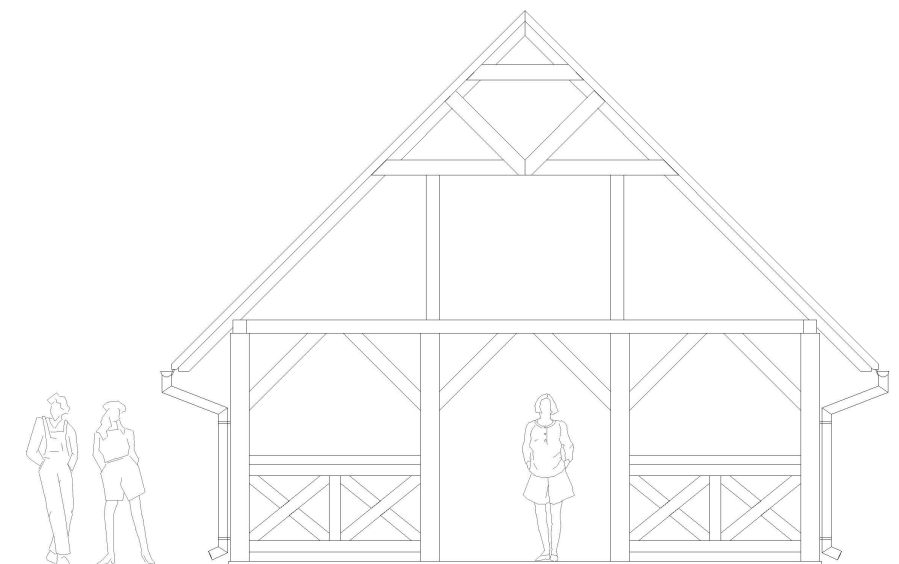
WIDOK PRZÓD
